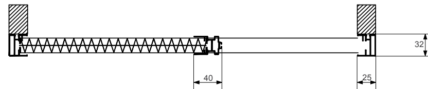
SEZ. ORIZZONTALE
