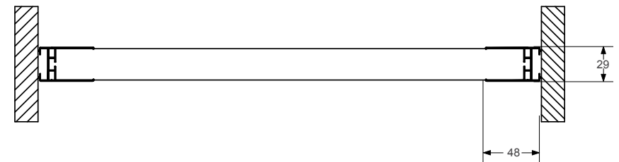
SEZ. ORIZZONTALE
