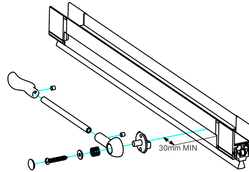
ASTA DA MONTARE SULLA BARRA MANIGLIA
