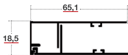
GUIDA CON TELAIO RINFORZATO
