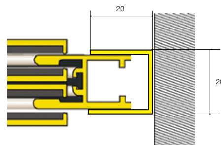
SEZ. ORIZZONTALE CON COMPENSATORE
