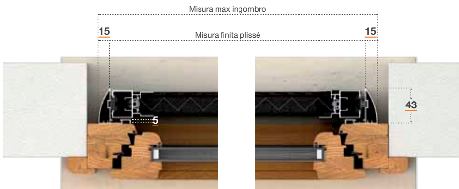
SEZ. ORIZZONTALE
